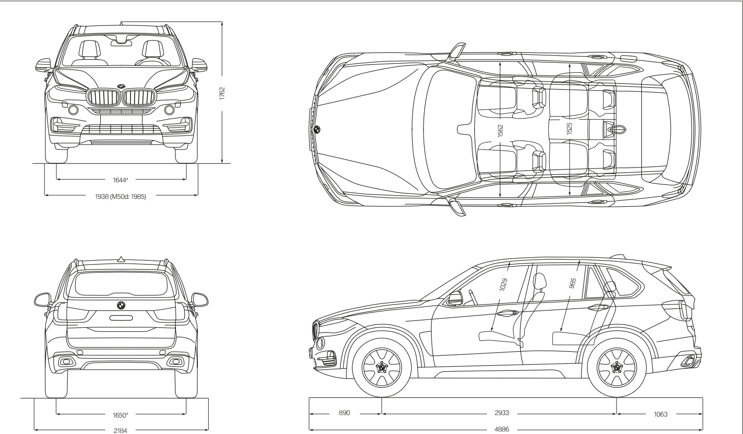
Alle Angaben der technischen Zeichnungen in Millimeter. Höhe mit Dachantenne angegeben.
